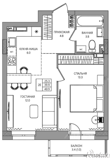
План 3-8 этажей
