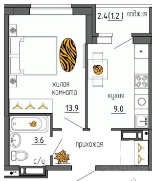
Корпус 1. План 3-15 этажей
